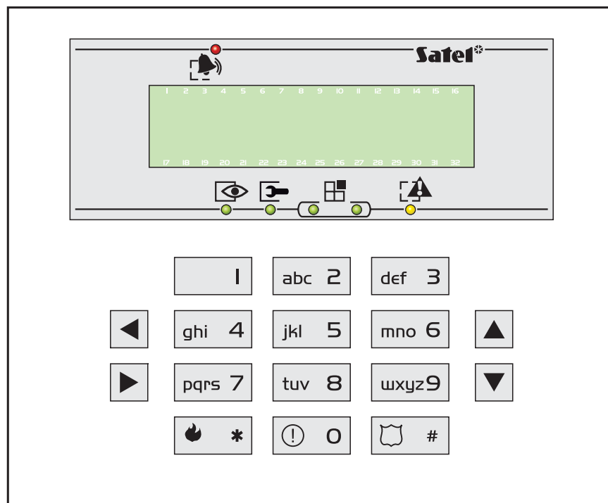
Rys. 2. Widok manipulatora INT-KLCDS-GR.
